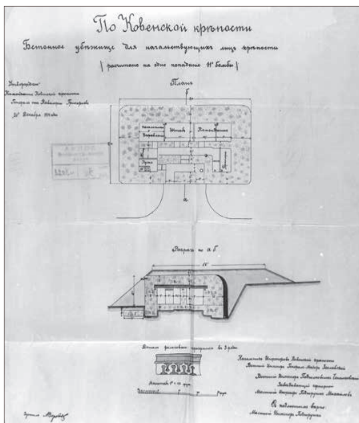
Kauno tvirtovės vadovybės betoninės slėptuvės projektas. 1914 m. VDKM negatyvų rinkiniai
