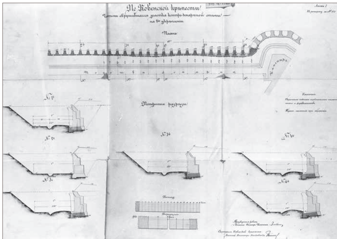
Kauno tvirtovės V forto sugriuvusios kontreskarpinės sienos brėžinys. XIX a. pab. VDKM negatyvų rinkiniai
