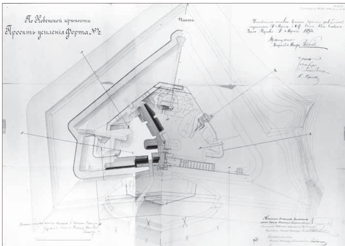
Kauno tvirtovės IV forto sustiprinimo projektas. 1893 m. VDKM negatyvų rinkiniai
