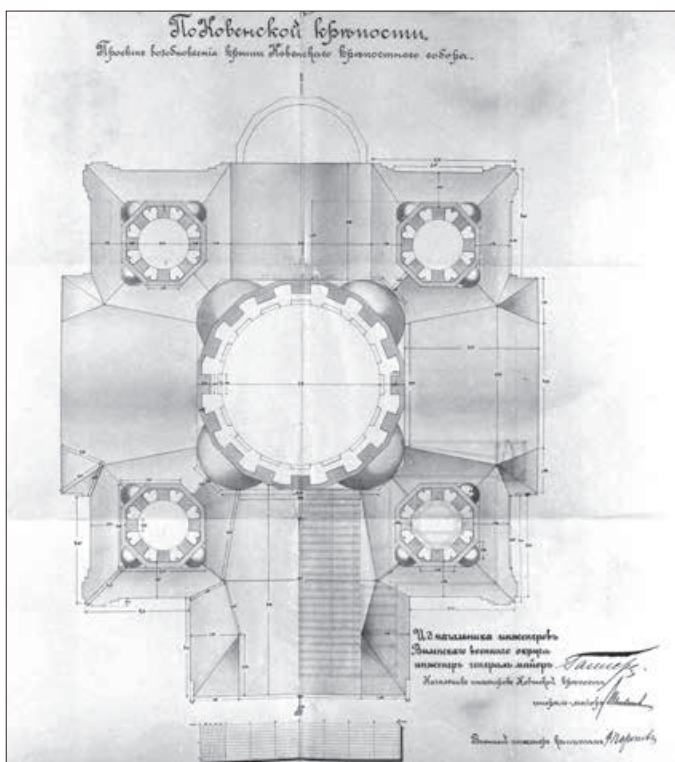
Šventųjų apaštalų Petro ir Povilo Kauno tvirtovės įgulos soboro pastato stogo atnaujinimo projektas. XX a. pr. VDKM negatyvų rinkiniai
