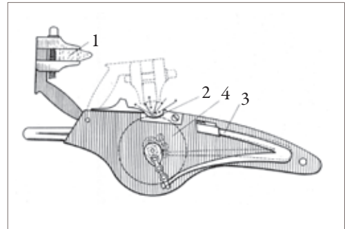
Ratukinės spynos veikimas. 1 – gaiduko laikomas piritas, 2 – parako lentynėlė, 3 – spyruoklė, 4 – ratukas
