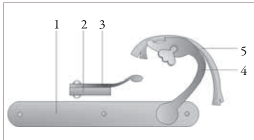
Dagtinė spyna. 1 – spynos plokštė, 2 – parako lentynėlė, 3 – lentynėlės dangtelis, 4 – serpentinas, 5 – dagtis
