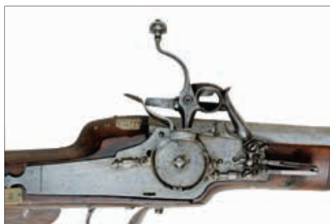
Ratukinės spynos vaizdas. Viršutinė gaiduko lūpa lenktu ūsu – rankenėle su profiliuotu rutuliu gale
