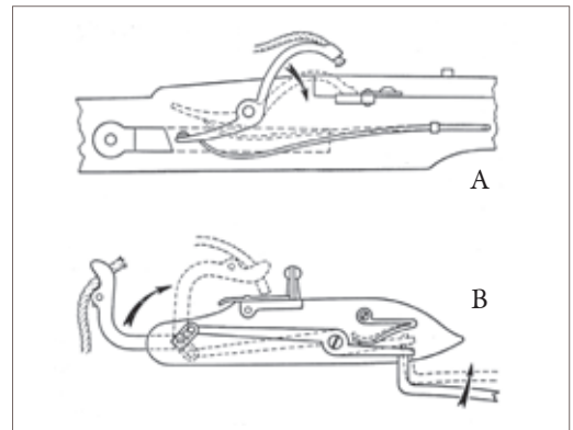
Dagtinės spynos veikimas: A – spyna spyruoklės judinamu serpentinu, XV a. pabaiga; B – spyna (vidinis vaizdas) svirtų judinamu serpentinu, XVI a. Iš leidinio: Жук А. Б. Стрелковое оружие. Москва, 1992
