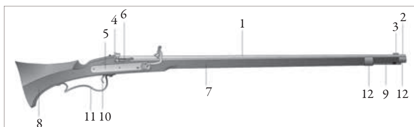
Muškieta dagtine spyna. 1 – vamzdis, 2 – laibgalis, 3 – kryptukas, 4 – taikiklis, 5 – spyna, 6 – parako lentynėlė ir dangtelis, 7 – apsodas, 8 – buožė, 9 – grūstuvai, 10 – nuleistukas, 11 – nuleistuko apsauga, 12 – apsodo apkaustai
