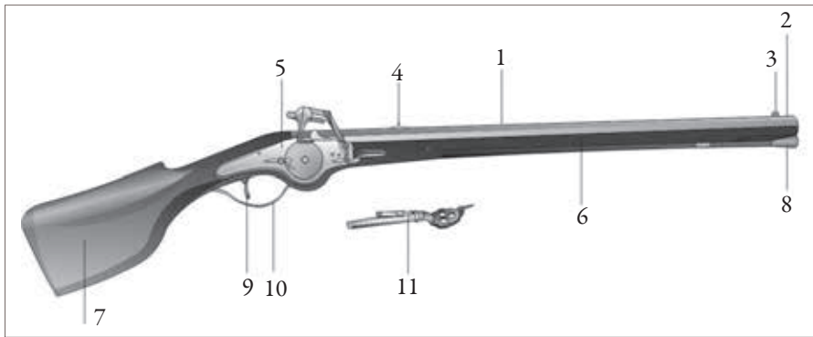
Šautuvas ratukine spyna. 1 – vamzdis, 2 – laibgalis, 3 – kryptukas, 4 – taikiklis, 5 – spyna, 6 – apšodas, 7 – buožė, 8 – grūstuvus, 9 – nuleistukas, 10 – nuleistuko apsauga, 11 – raktas spynos mechanizmui prisukti
