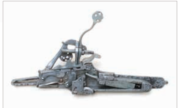
Šautuvo ratukinės spynos vidinė pusė. Europa, XVII a.
