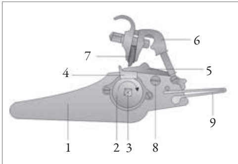
Ratukinė spyna. 1 – spynos plokštė, 2 – ratukas, 3 – ratuko ašis, 4 – parako lentynėlė, 5 – lentynėlės dangtelis, 6 – gaidukas, 7 – piritas, 8 – lentynėlės dangtelio varžtas, 9 – gaiduko spyruoklė
