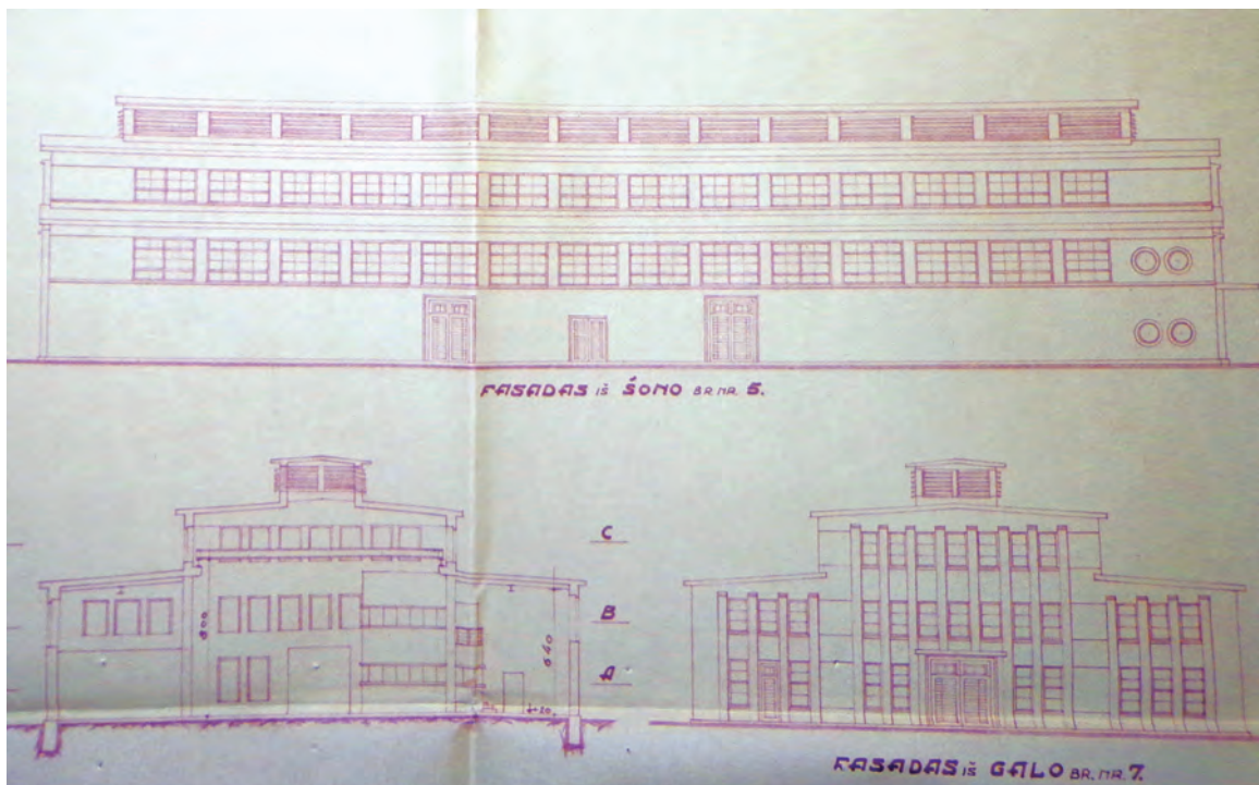
Ginklavimo valdybos civilinio tarnautojo architekto B. Elsbergo suprojektuoto Linkaičių ginklų dirbtuvių Artilerijos skyriaus pastato H fasado brėžinys.
