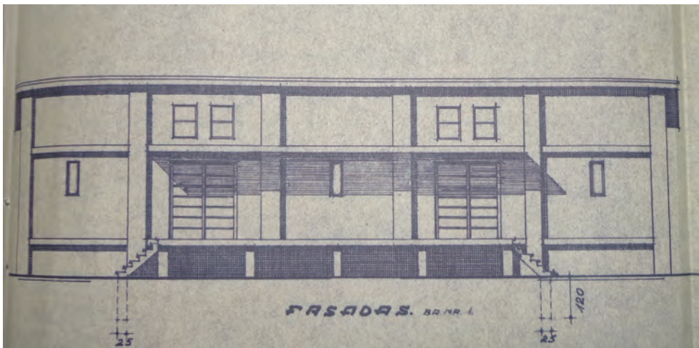
Ginklavimo valdybos civ. tarnautojo architekto Broniaus Elsbergo projektuoto Linkaičių artilerijos sandėlio „A“ fasado brėžinys. 1936 m.
