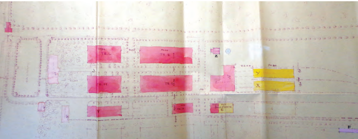
Ginklavimo valdybos civ. tarnautojo architekto B. Elsbergo sudaryto Linkaičių artilerijos dirbtuvių situacijos plano dalis. 1937 m. birželio 7 d. plane pavaizduotas pastatų išsidėstymas teritorijoje. Raudona spalva pažymėti pastatyti arba dar statomi mūriniai pastatai. Rožine spalva pažymėti planuojami statyti mūriniai pastatai. Geltona spalva pažymėti planuojami statyti mediniai pastatai.
